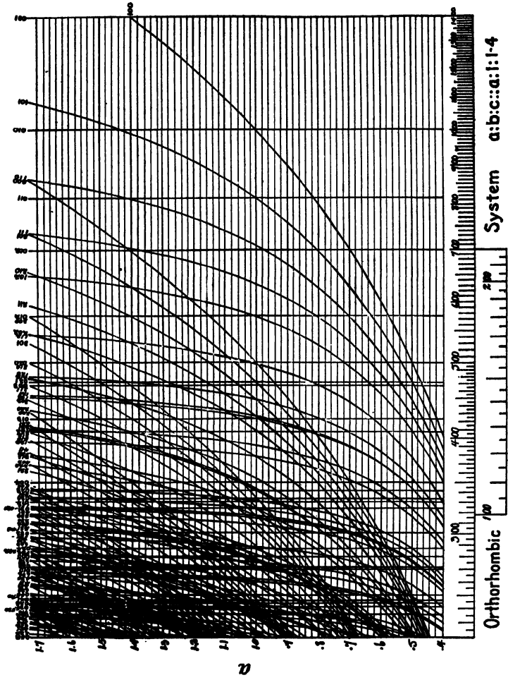
FIG. 17.—Orthorhombic system, a:b:c::a:1:4 .
